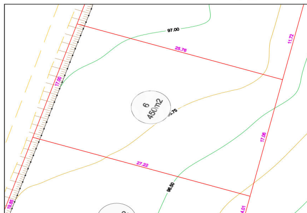
PLAN FONCIER DU LOT Echelle : 1/200
