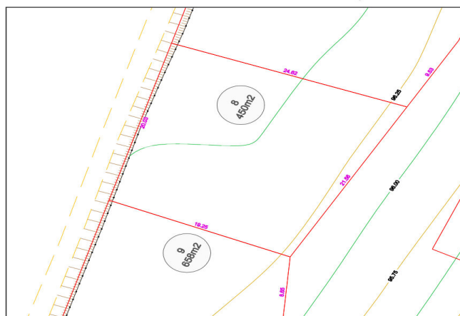
PLAN FONCIER DU LOT Echelle : 1/250
